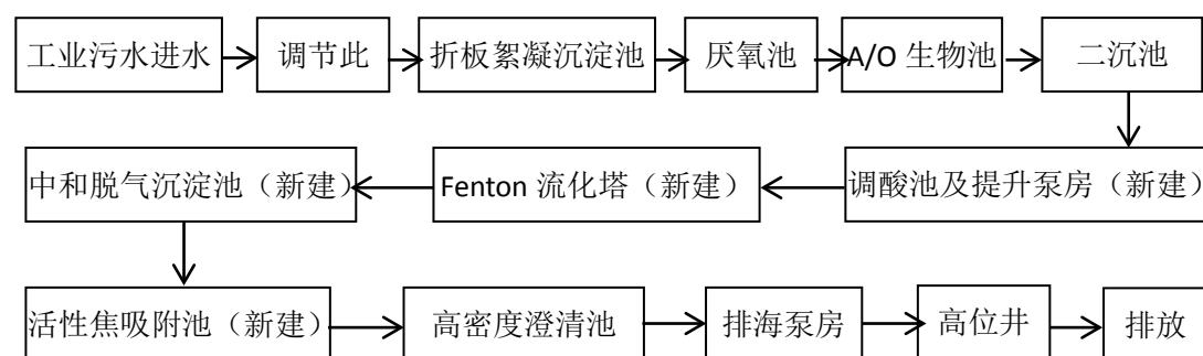
图 2-3 上虞污水处理厂提标改造工程工业污水处理工艺流程图
