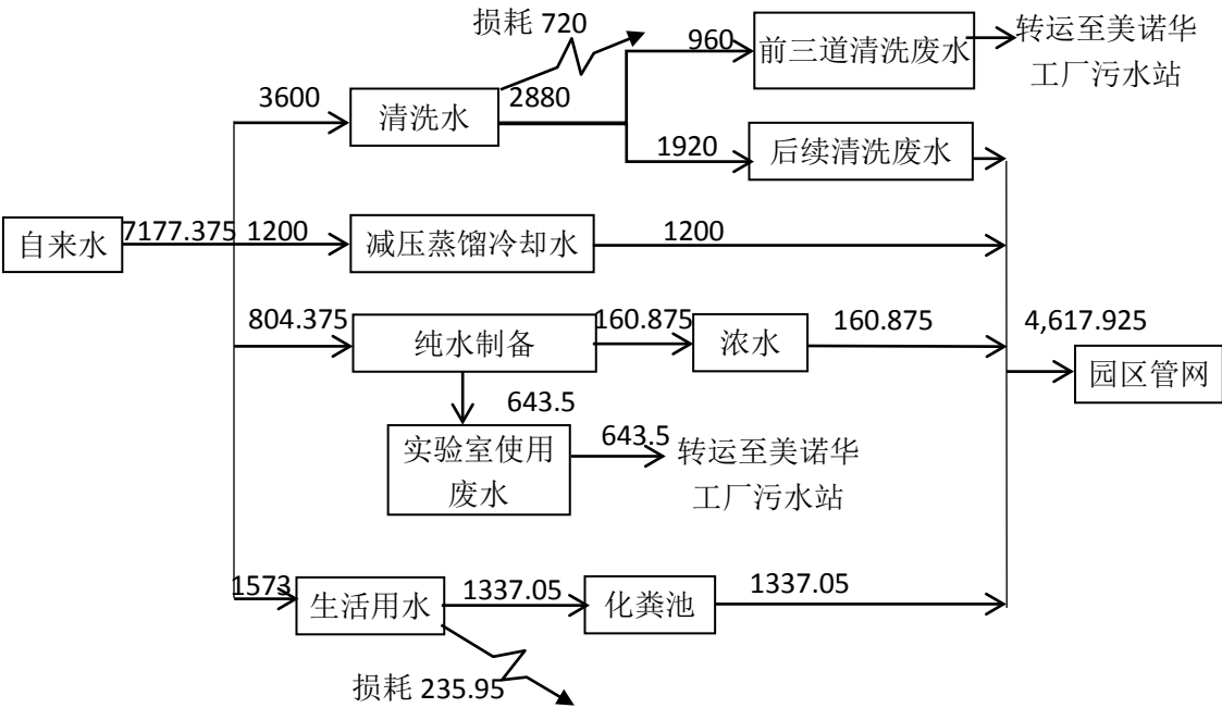
图 5-2 项目运营期水平衡图（单位：t/a）
