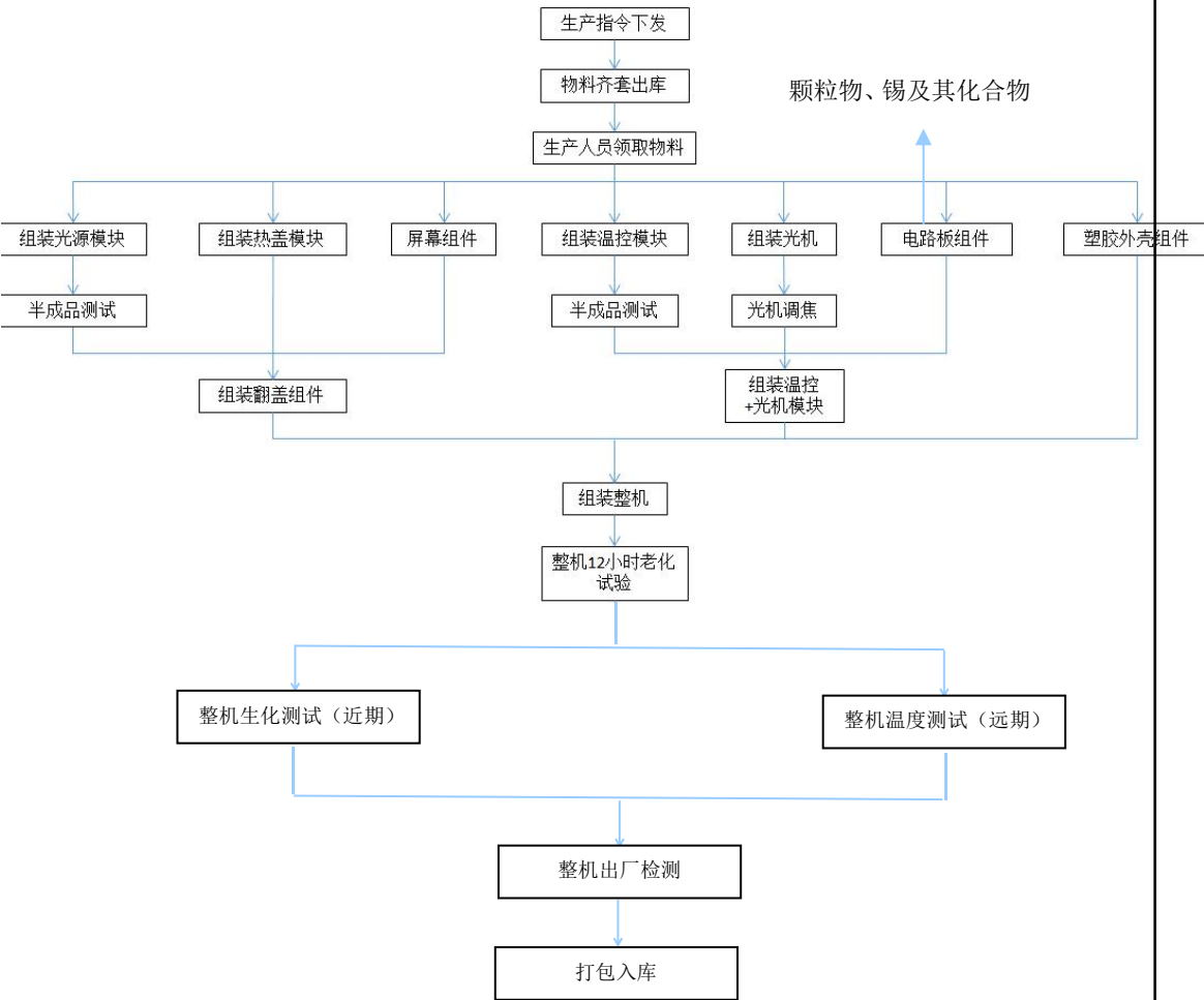
图 5-1 生产工艺流程图
